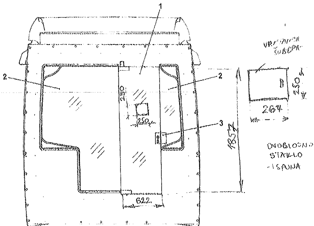
Slika 3-11. Vrata između kabine i salona
